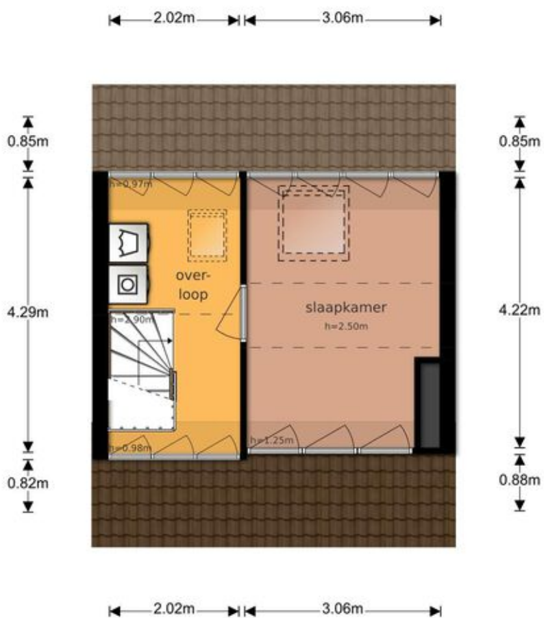
Venderinklanden 5 - Enschede Tweede Verdieping
